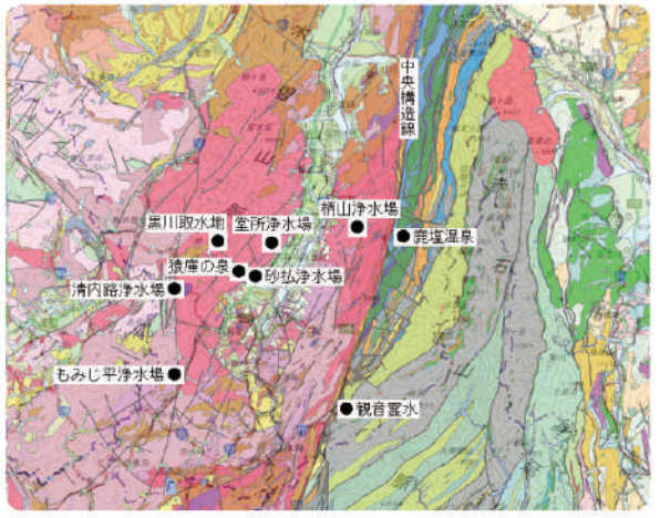
伊那谷の地質図。赤・ピンク色が花崗岩質のエリア(地質図Navi https://gbank.gsj.jp/geonavi/ の画像を加工)
